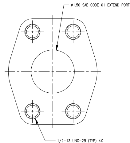
DETAIL A-A SCALE 1:1
